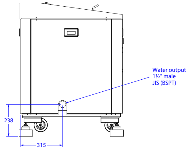
Left
